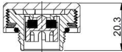
A-A (1 : 1)
